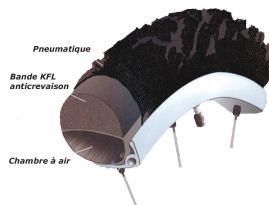
BANDE ANTI-CREVAISON KFL
